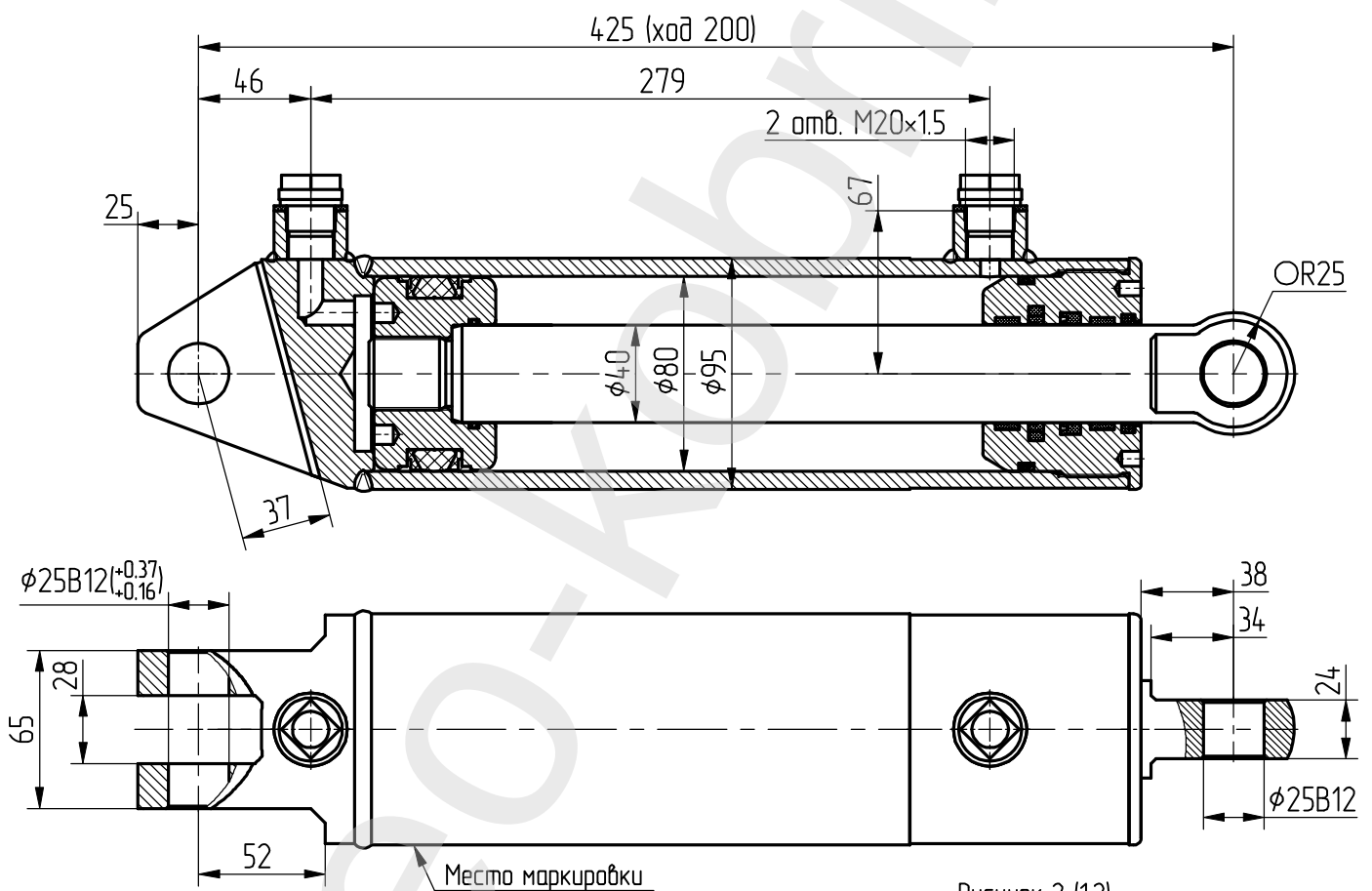
Рисунок 2 (1:2) Остальное-смотри рисунок 1
