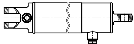
Рисунок 3 (1:2) Остальное-смотри рисунок 1
