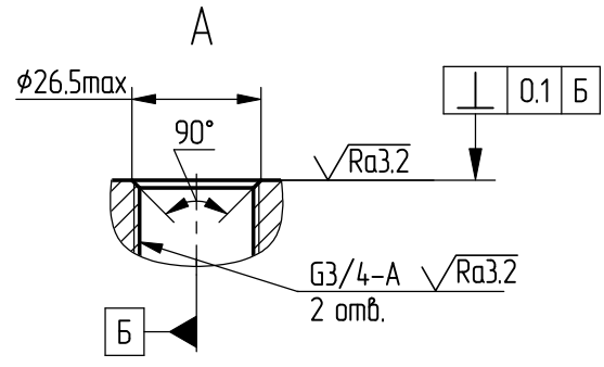
Рисунок 3 Остальное - смотри рисунок 1 (для исполнения -02) или рисунок 2 (для исполнения -03)
