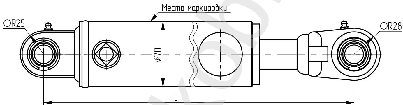
Остальное – смотри рисунок 1 М (1:2)
