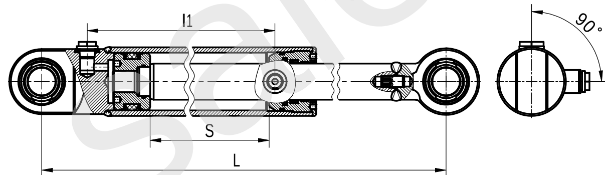
Рисунок 3 (1:2) Остальное - см. рисунок 1
