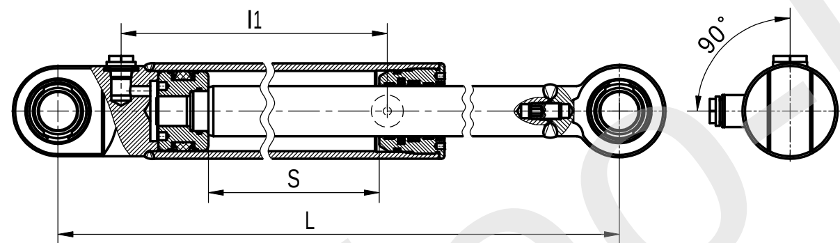
Рисунок 2 (1:2) Остальное - см. рисунок 1
