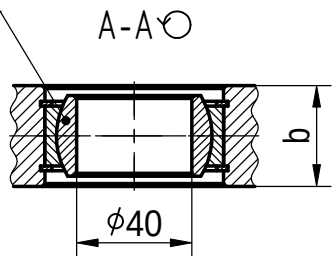
Подшипник GE40ES ISO 12240-1 2 шт.
